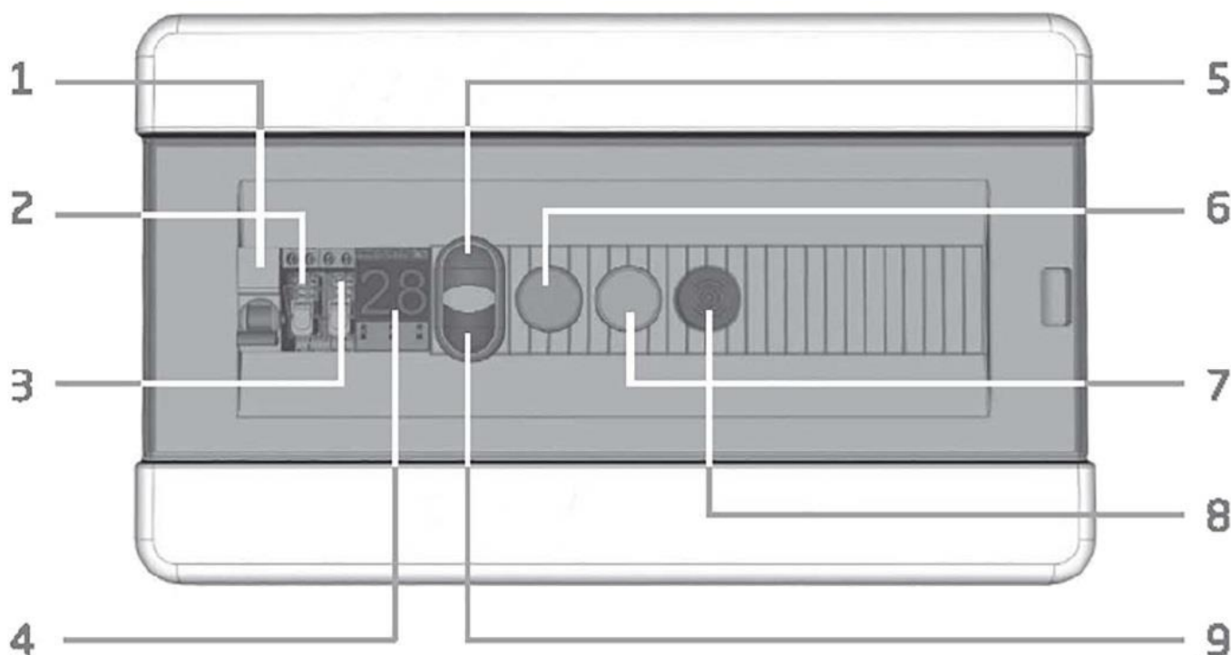
Рис. 1. – Щит управления
